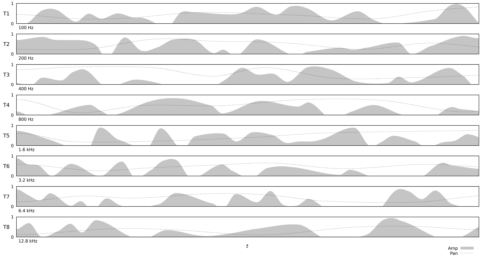
Amplitudenverlauf der 8 Bandpässe ( Q = 1.414 ) und deren Spatialisation (0.5 = Front center, 0.0/1.0 = Back center)
